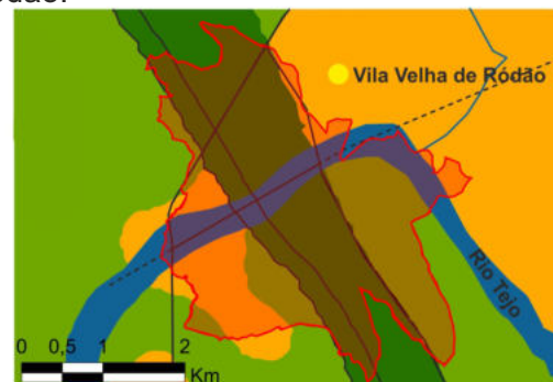
Mapa geológico geral do MNPR
